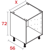
Módulo Cajonero B72
