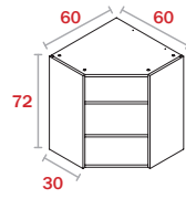
Módulo Chafián H72
