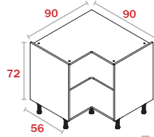
Módulo Esquina "L" B72
