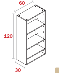
Módulo Sobre Encimera H120
