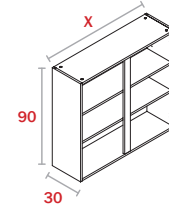
Módulo Superior Doble H90
