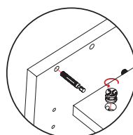
Montaje con excéntrica y perno expansible
