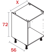
Módulo Cajon+Puerta B72
