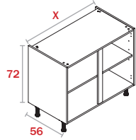
Módulo Inferior Doble B72
