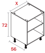
Módulo Inferior Simple B72
