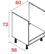
Módulo Horno B72
