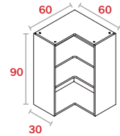
Módulo Esquina "L" H90
