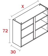
Módulo Superior Doble H72
