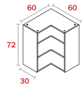
Módulo Esquina "L" H72
