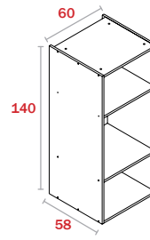
Semicolumna
